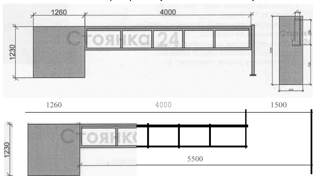
Технические характеристики устанавливаемого шлагбаума
