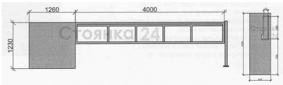
Технические характеристики устанавливаемого шлагбаума
